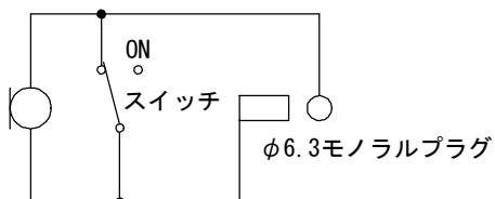
接続図
